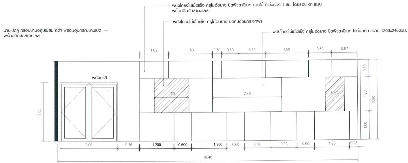
W1 รูปด้าน ห้องคอมพิวเตอร์
