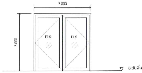
D2 ประตูอลูมิเนียมบานเปิดคู่
