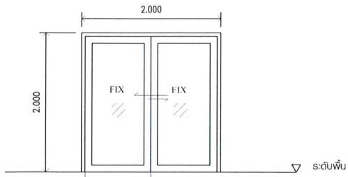
D1 ประตูอลูมิเนียมบานเลื่อนคู่
