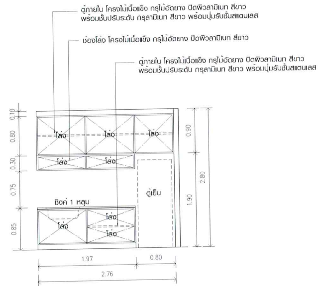
B3 รูปด้านในเคาน์เตอร์ ชุด Pantry
