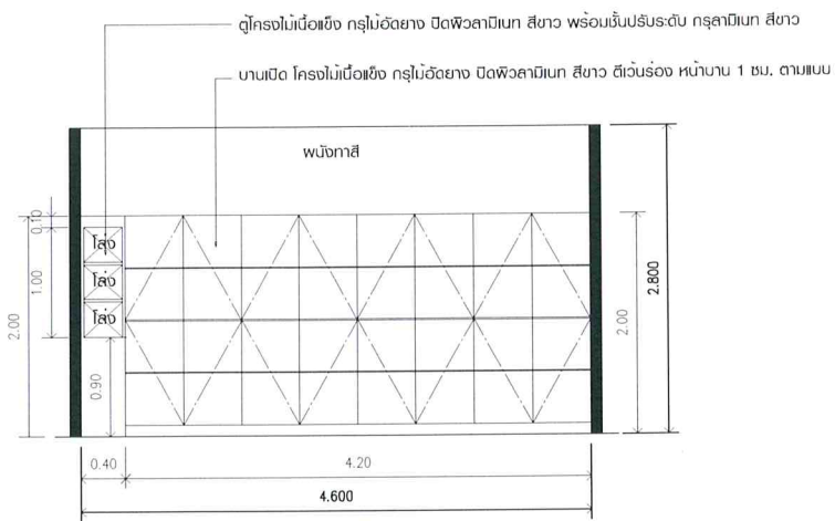
B2 รูปด้าน ตู้ออกสาร / ตูเก็บชุด
