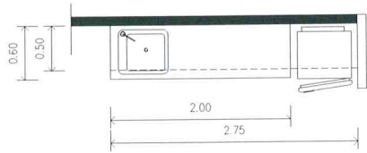
B3 แปลนเคาน์เตอร์ ชุด Pantry
