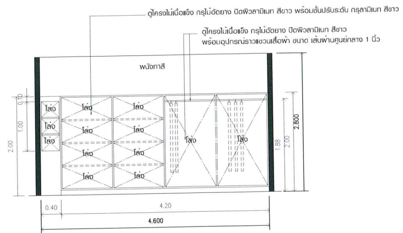
B2 รูปด้านใน ตู้ออกสาร / ตูเก็บชุด
