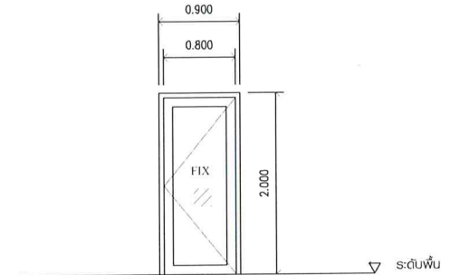
D3 ประตูอลูมิเนียมบานเปิดเดี่ยว
