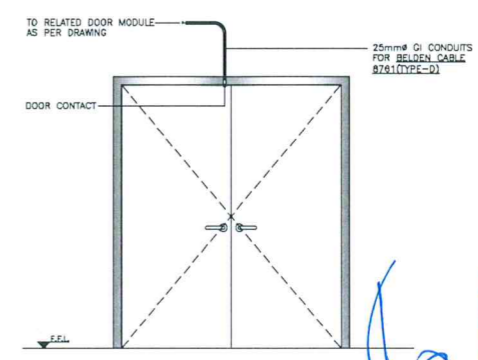
DETAIL FOR DOUBLE DOOR TYPE-2 SCALE: N.T.S.
