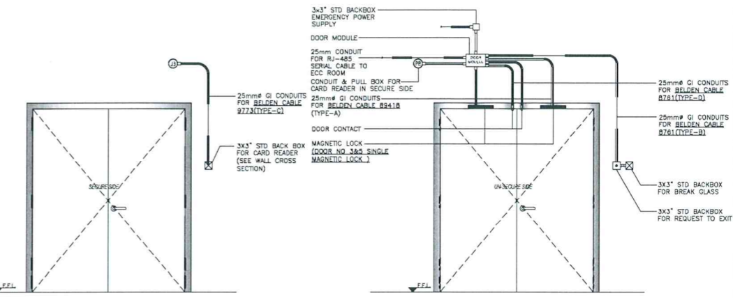
DETAIL FOR DOUBLE DOOR TYPE-1 SCALE: N.T.S.
